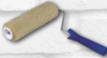
RODILLO DE HILO PARA SUPERFICIES RUGOSAS 220 MM Ø45 MM Ref: 15005530
